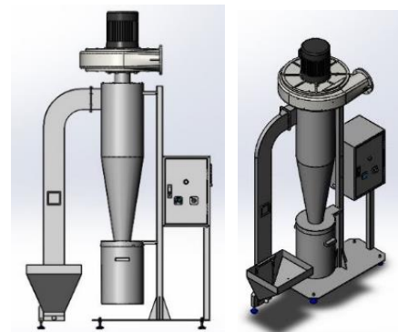
Gambar 2. Konsep Desain Destoner Kopi
