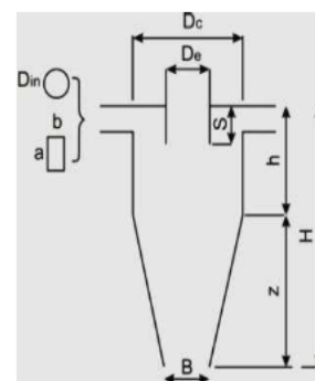
Gambar 6. Variasi Dimensi
