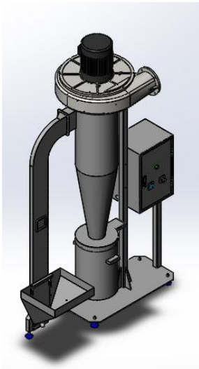
Gambar 15. Desain Mesin Destoner Kopi
