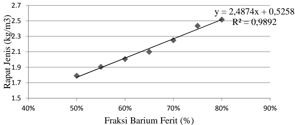
Gambar 3. Grafik hubungan antara fraksi barium ferit dengan rapat jenis.
