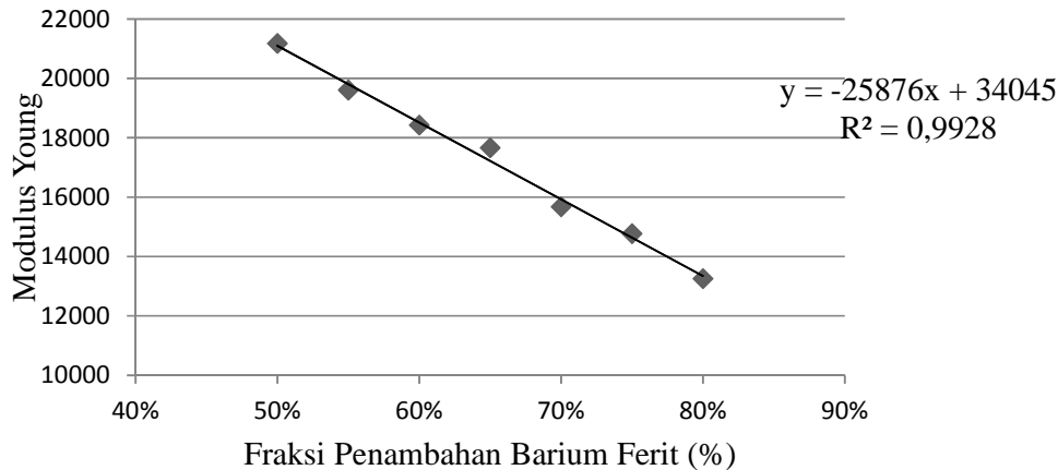
Gambar 1. Hubungan antara besar komposisi barium ferit dengan modulus Young.
