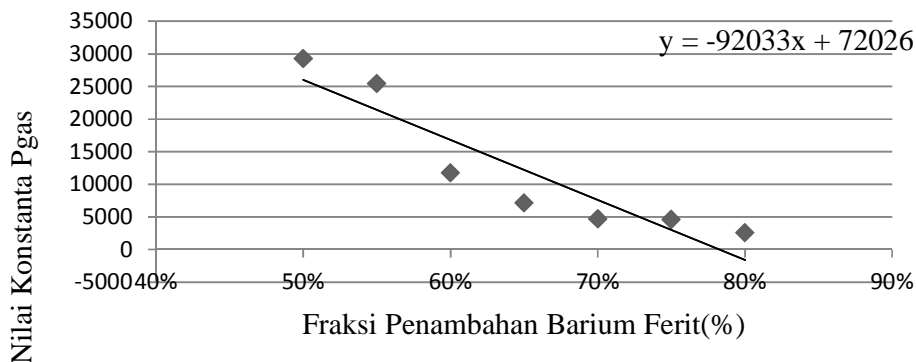
Gambar 2. Grafik hubungan antara fraksi barium ferit dengan konstanta pegas rata-rata.
