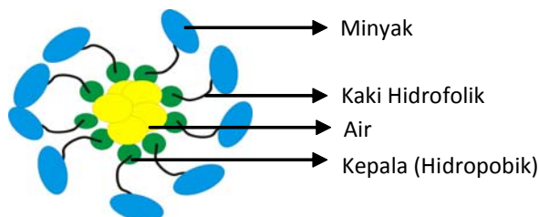
Gambar 3. Ikatan Molekul Minyak dan Air
