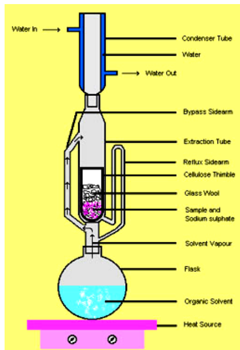
Gambar 2. Ekstraksi Soxhlet
