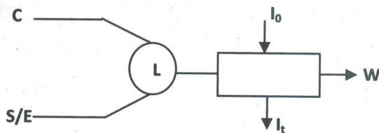
Gambar 4. Skema Sistem FIA Penelitian
