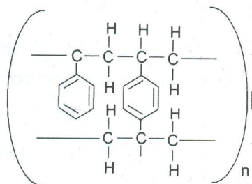
Gambar 2. Struktur Amberlite® Resin XAD-4
