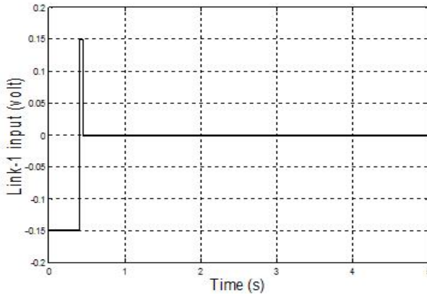
Gambar 2. Input Bang-bang
